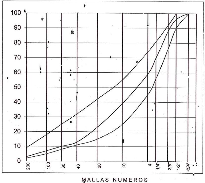
GRÁFICA DE COMPOSICIÓN GRANULOMÉTRICA
